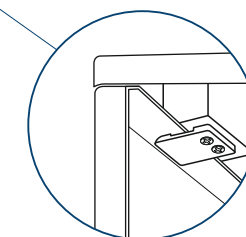
УЛУЧШЕННЫЙ ВАРИАНТ КРЕПЛЕНИЯ ЭКРАНА К БОРТАМ ВАННЫ
