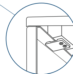
УЛУЧШЕННЫЙ ВАРИАНТ КРЕПЛЕНИЯ ЭКРАНА К БОРТАМ ВАННЫ
